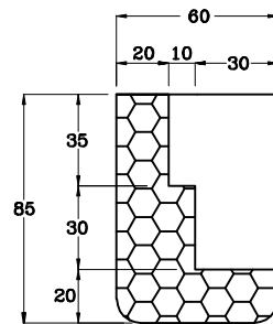
SEZ. B-B
