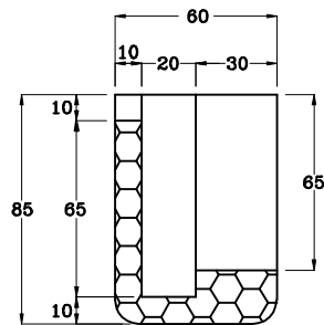
SEZ. A-A
